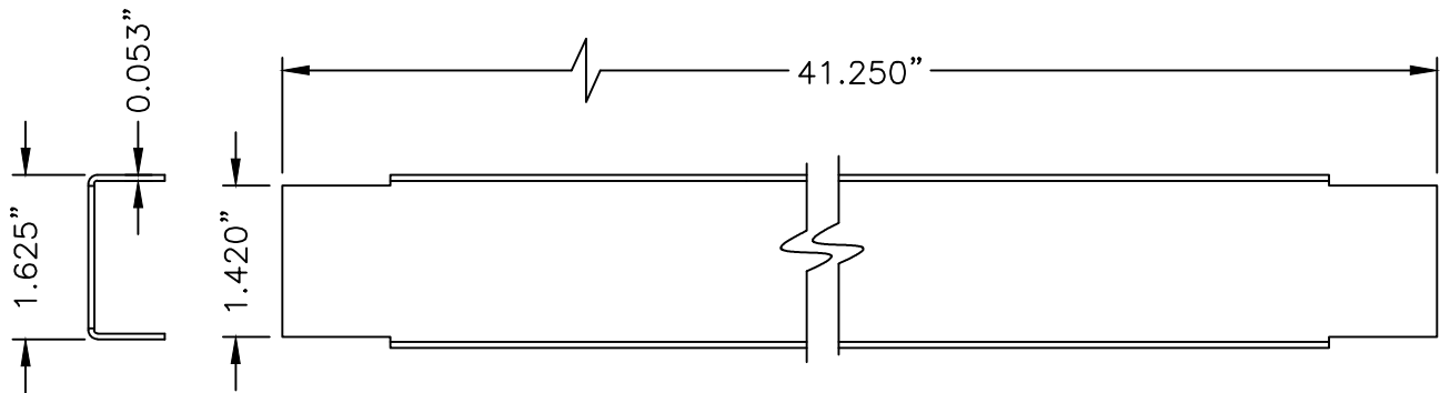
13 DOOR TOP & BOTTOM CLOSER 16GA. (.053) C.R.S.
